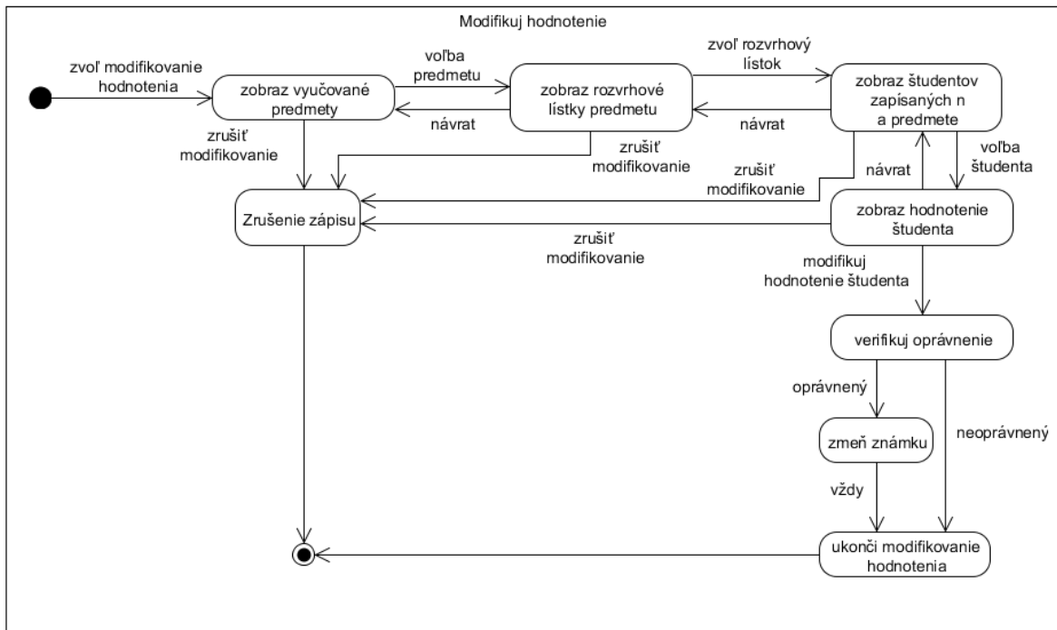
Obrázok 2:Stavový Diagram
