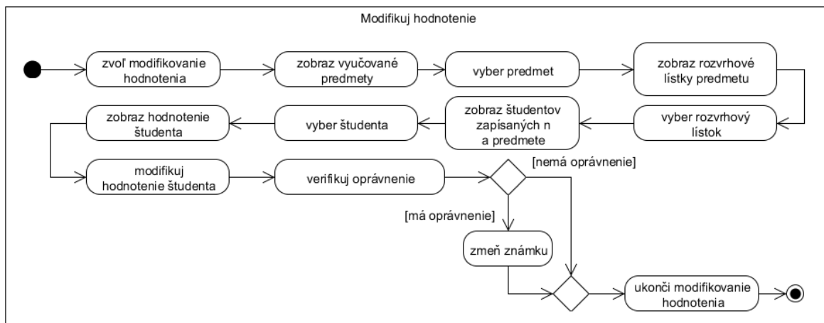
Obrázok 1:Aktivity Diagram
