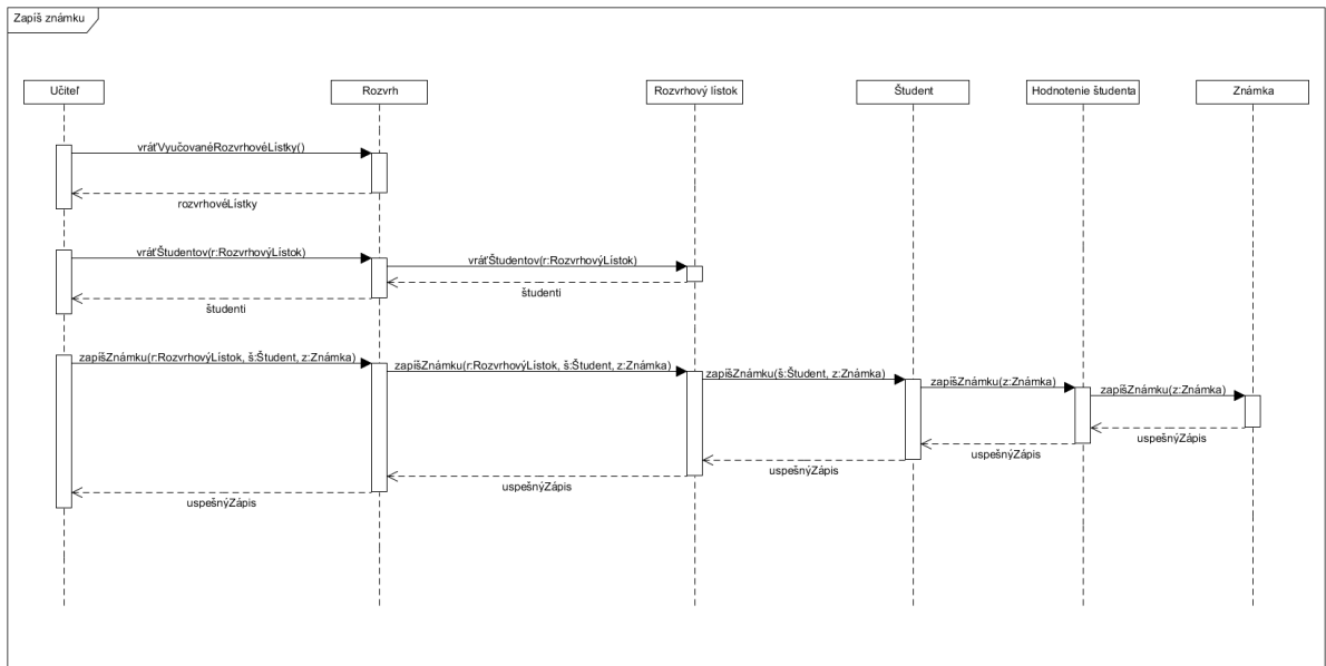
Obrázok 3: Sekvenčný Diagram
