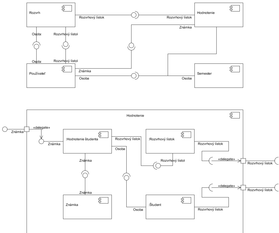
Obrázok 2: Komponent diagram
