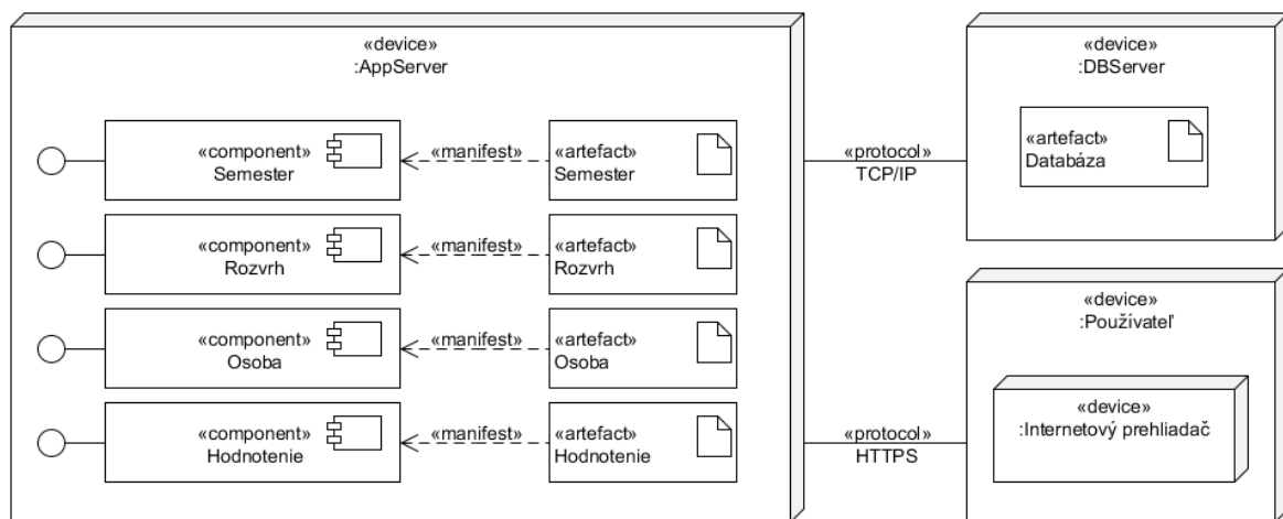
Obrázok 3: Deployment diagram
